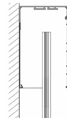
TYP C - Kasten für Fassadenmontage. Passende Führungsschienen F-FBR-010.
