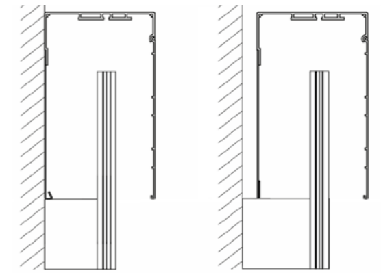
TYP C - Kasten für Fassadenmontage. Passende Führungsschienen F-FBR-010.
