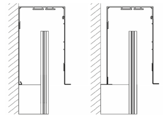
TYP A - Einbaukasten. Passende Führungsschienen F-FBR-030. TYP B - Einbaukasten, abgesetzt. Passende Führungsschienen F-FBR-040.
