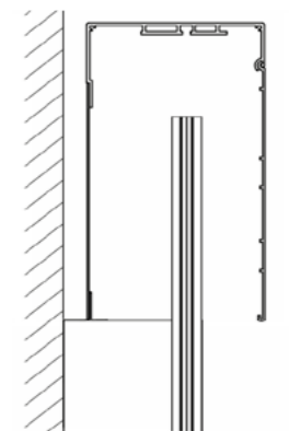
TYP D - Kasten für Fassadenmontage, abgesetzt. Passende Führungsschienen F-FBR-020.
