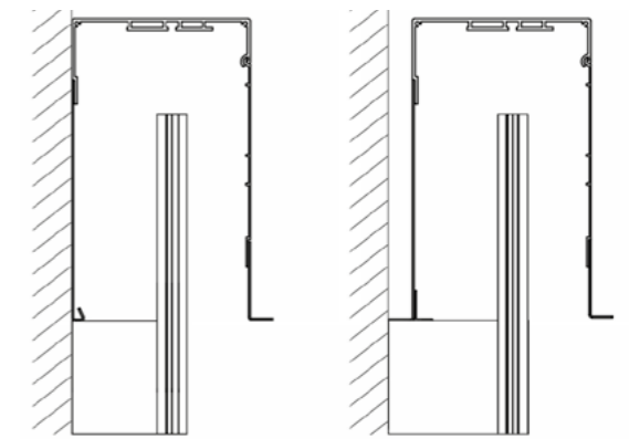
TYP A - Einbaukasten. Passende Führungsschienen F-FBR-030.
